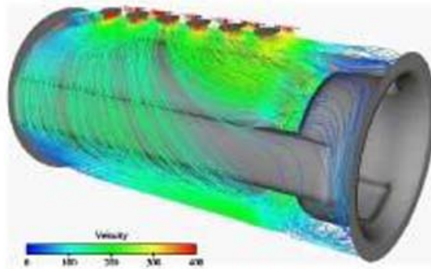
案例6: TRW的安全气囊气体发生器耦合分析
