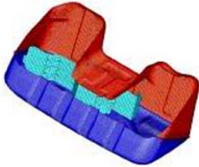
案例6: TRW的安全气囊气体发生器耦合分析
