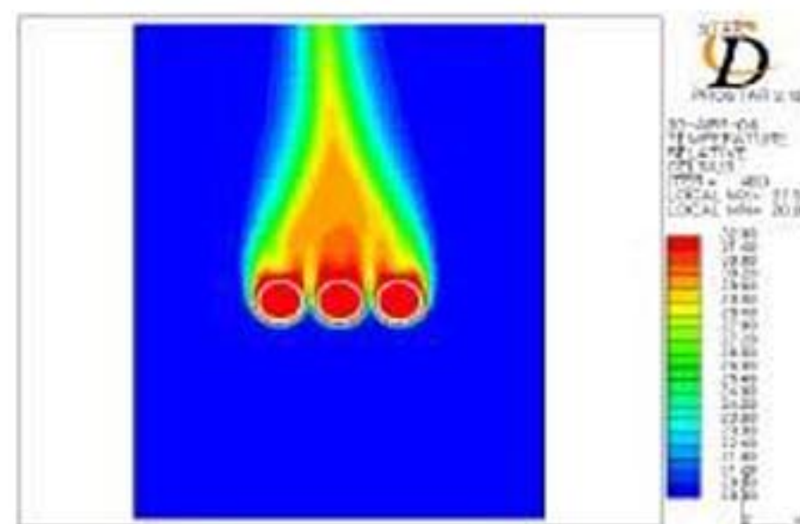
案例12：激光切削过程的耦合分析
