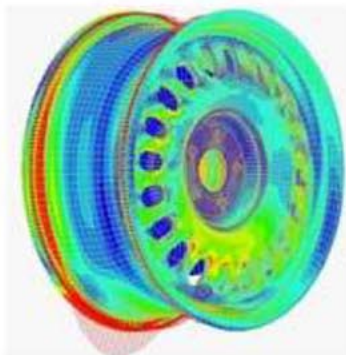
案例8: 高频载荷或高温条件下的疲劳寿命预报
