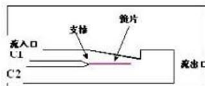
案例13：空调压缩机压力阀的耦合分析
