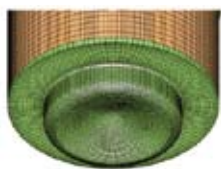
外部生成网格与模板结合（左为燃烧室，右为气道）
