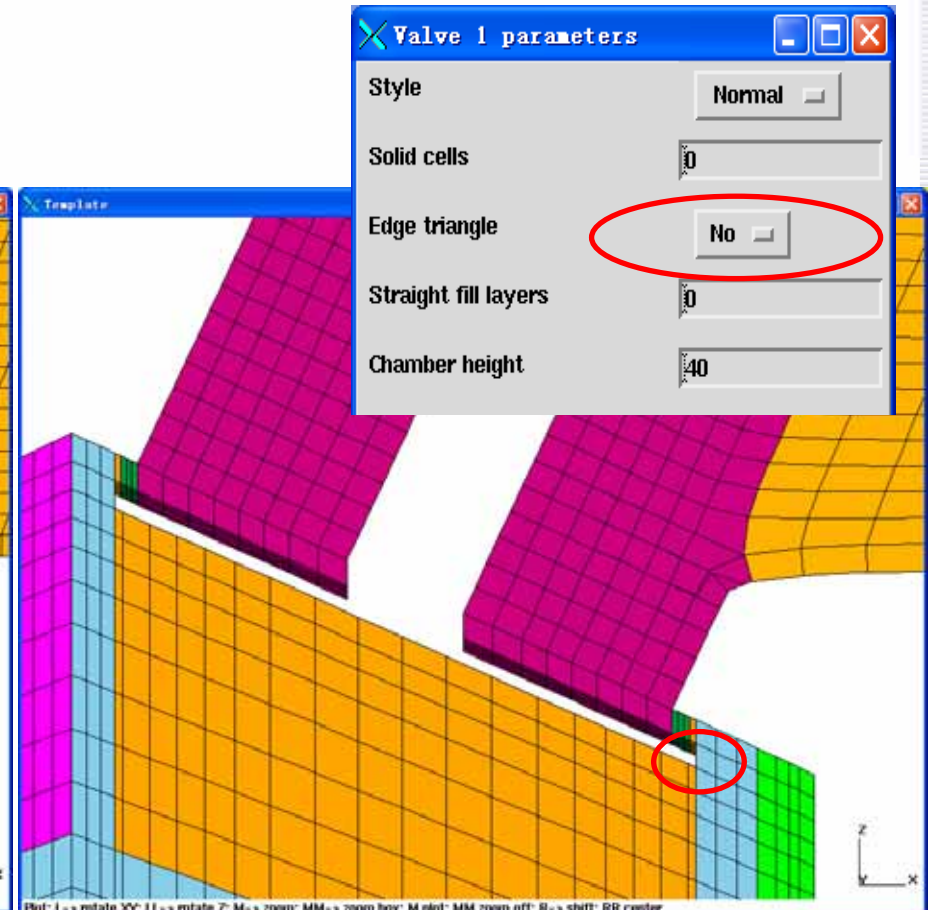
特殊气阀
