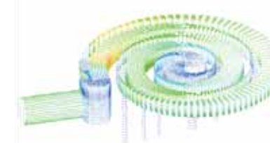
涡旋压缩机解析速度场
