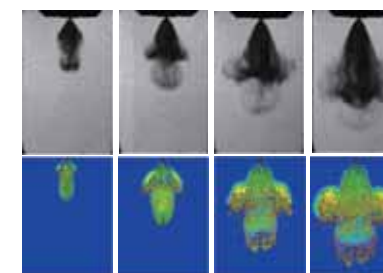
定容弹喷油实验与 STAR-CD计算结果对比
