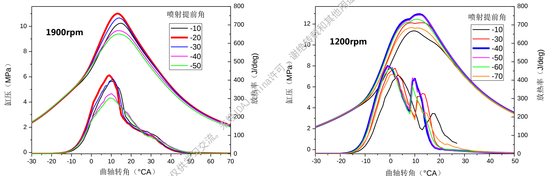
不同喷射正时的缸压及放热率（框选表示混合均匀度最好的工况）
