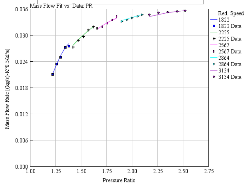
GT-SUITE涡轮MAP
